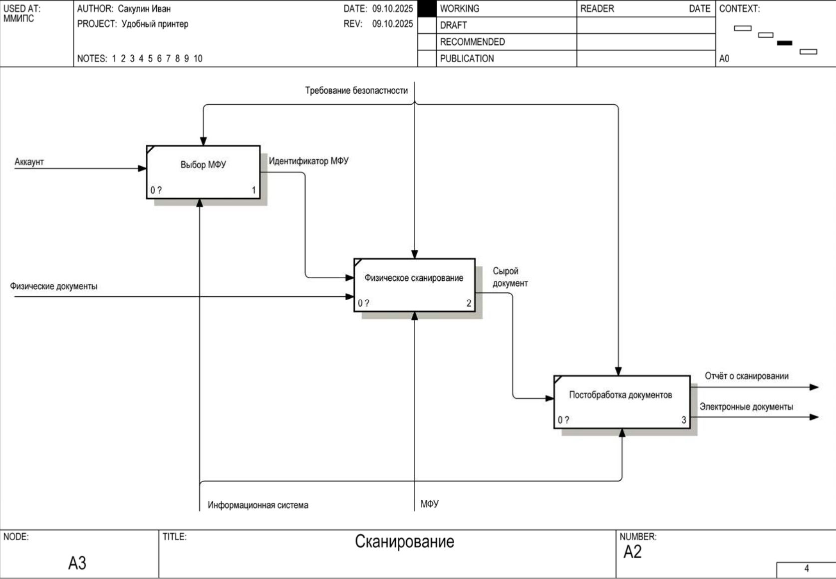
Рисунок 4 — Декомпозиция процесса «Сканирование» A2
