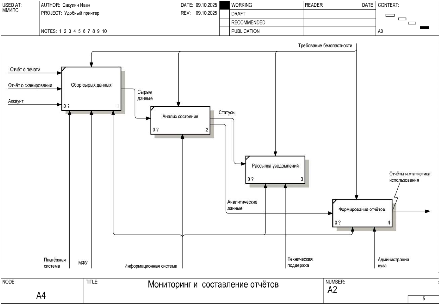
Рисунок 5 — Декомпозиция процесса «Мониторинг» A2
