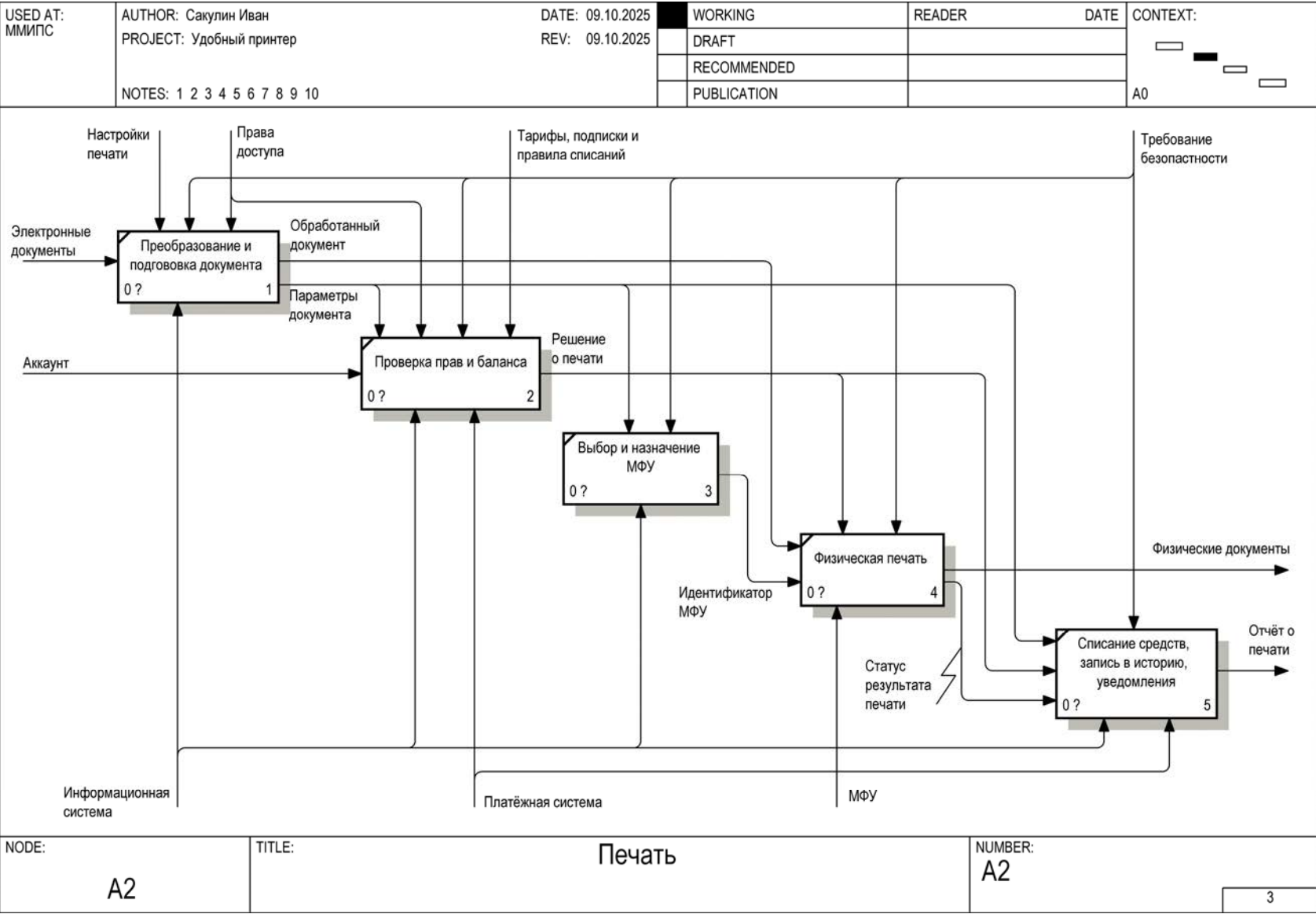
Рисунок 3 — Декомпозиция процесса «Печать» A2
