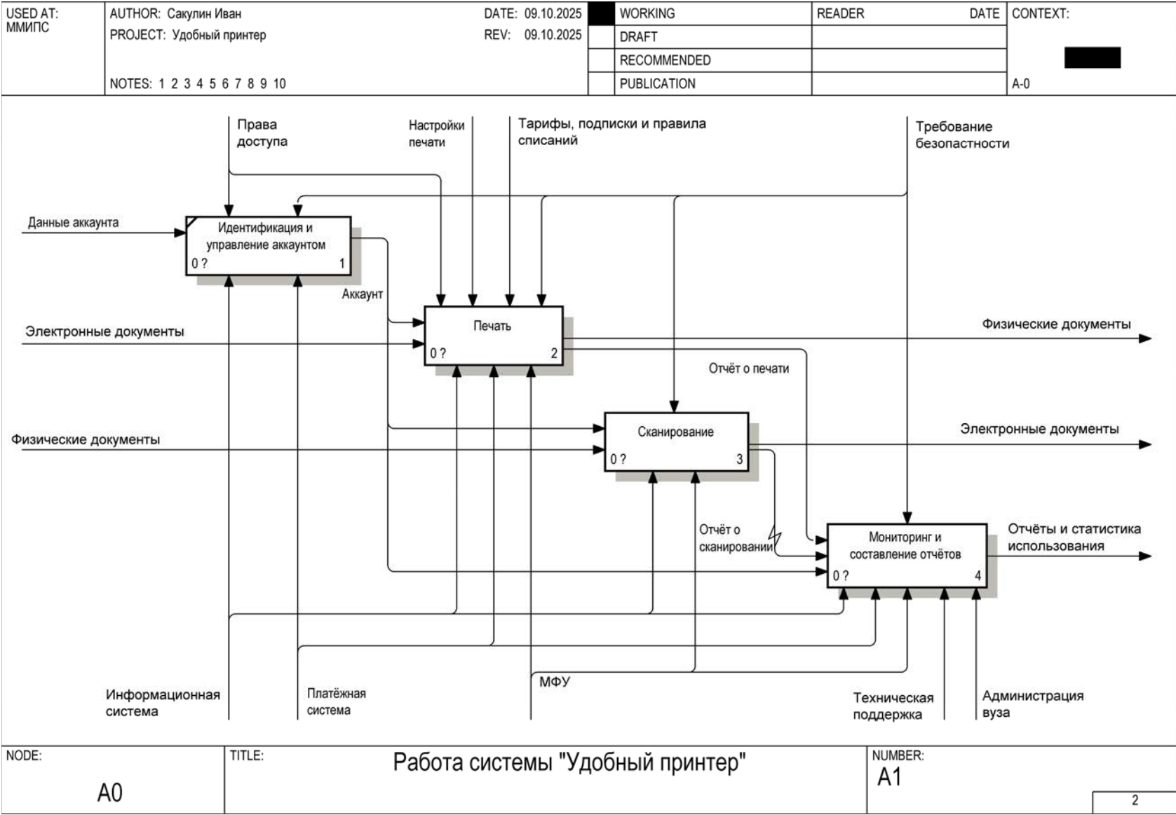
Рисунок 2 — Декомпозиция контекстной диаграммы A1
